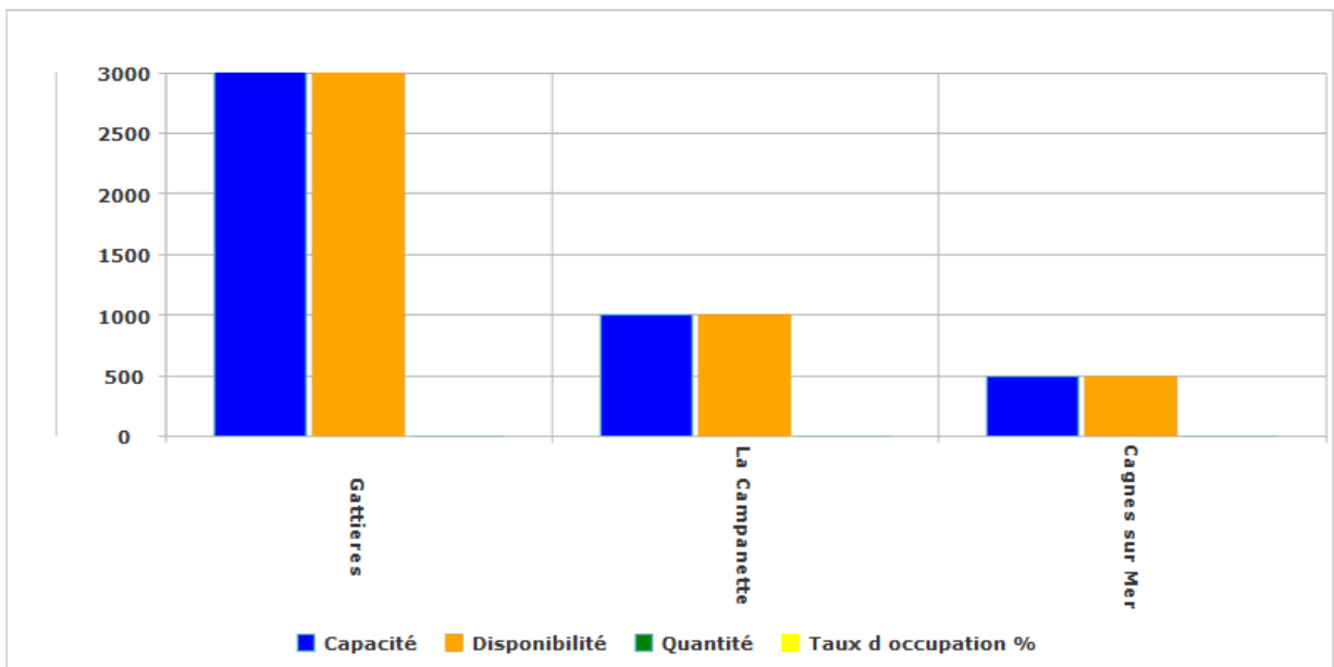
Figure 3 : statistiques générales
