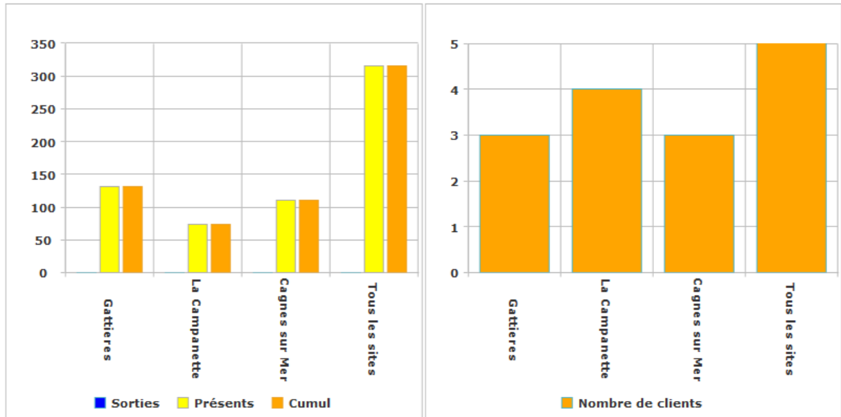
Figure 2: statistiques générales
